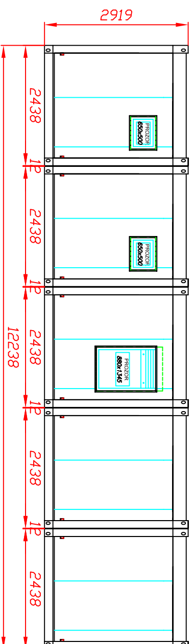
ANSICHT "D"
